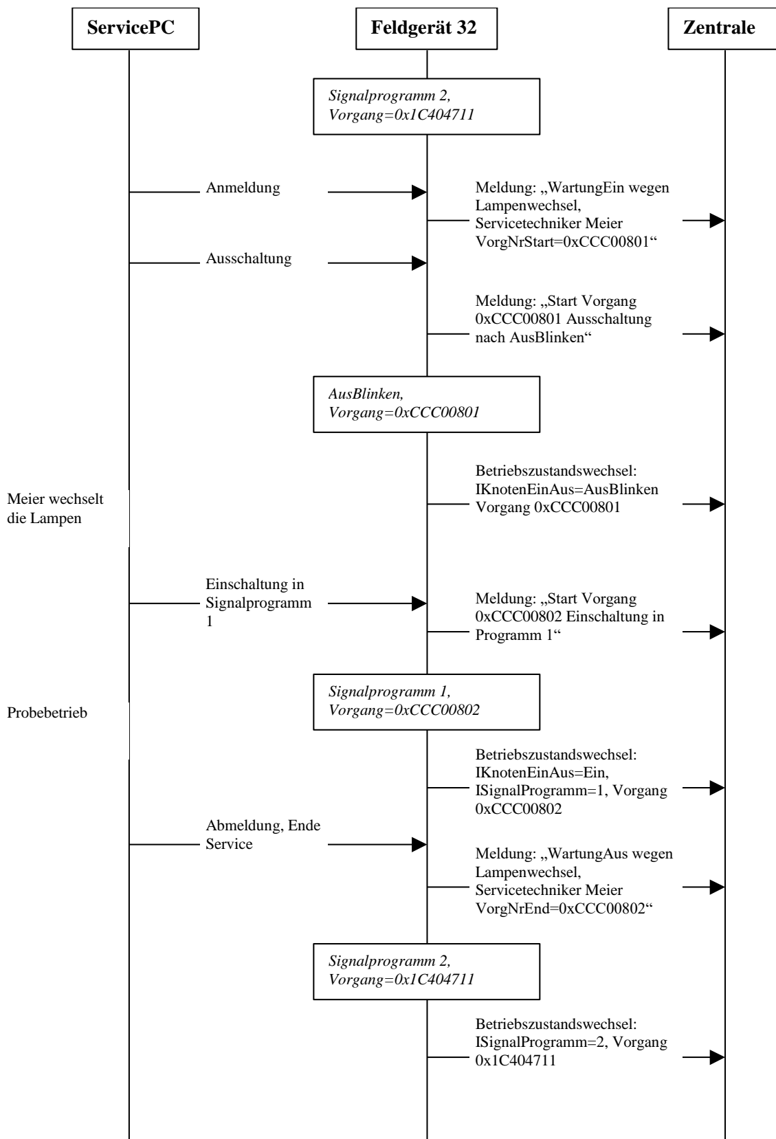
Abbildung 1: Ablaufschema zum Beispiel Lampenwechsel
