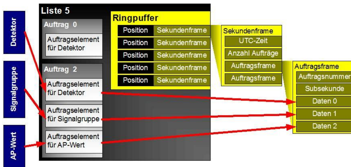
Abbildung 3: Schema einer Liste
