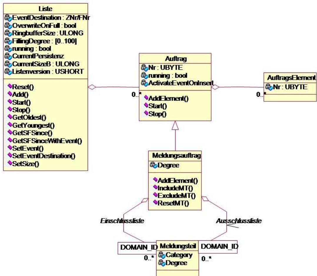
Abbildung 2: Schema der Archivschnittstelle
