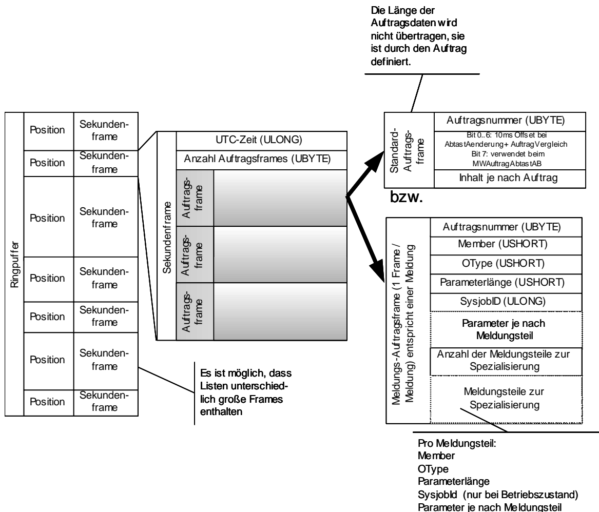
Abbildung 4: Schema Sekunden- und Auftragsframe
