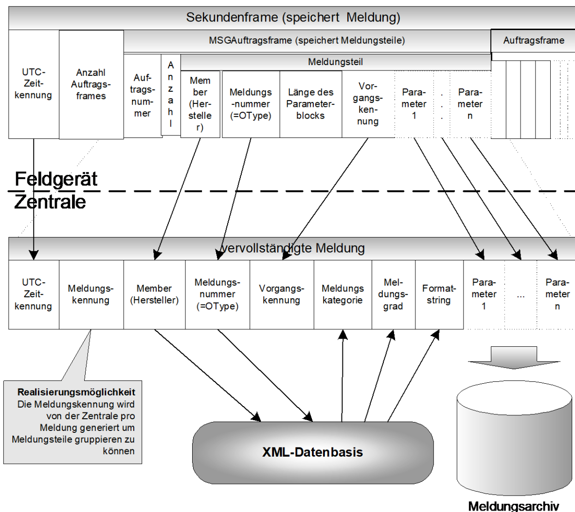
Abbildung 5: Schema der Handhabung von Meldungen
